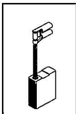
KBHLAGE2423C 6 x 16 x 20 mm.
