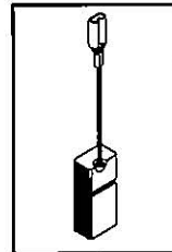
KBBOS918 5 x 8 x 17 mm.
